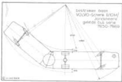
Ruimtebeslag voertuig versus draaicirkel assen
